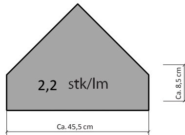
Fot/mønestein
