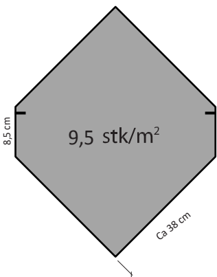
Firkantstein
